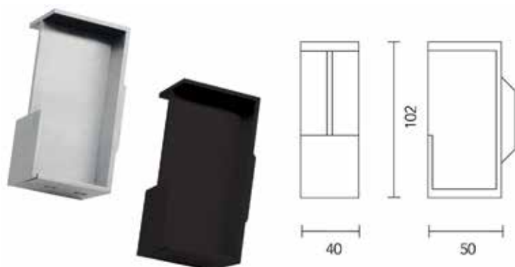
Poignée pour porte coulissante Carré massif - matière première: inox AISI 304
