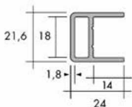
profil de renforcement profil-poignée
