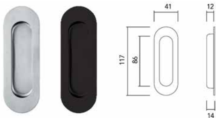
Poignée pour porte coulissante Oval aveugle - matière première: inox AISI 304
