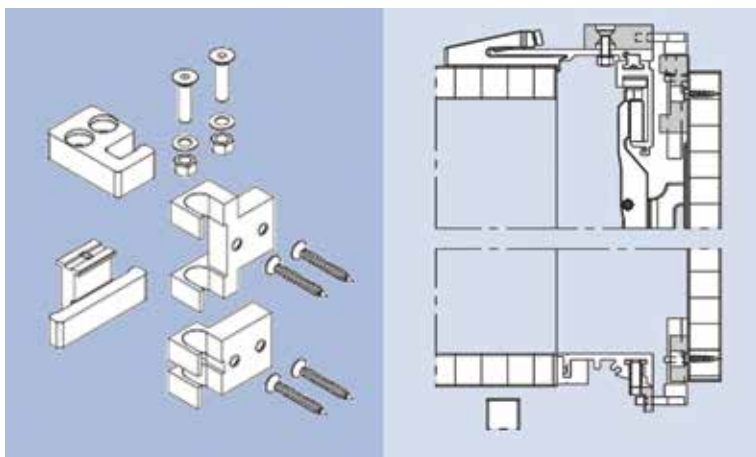
Kit de gâche pour serrure à tringle pour Hawa Folding Concepta 25 - kit pour 1 porte
